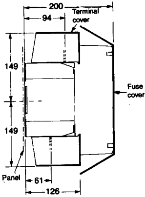
UFS 315
